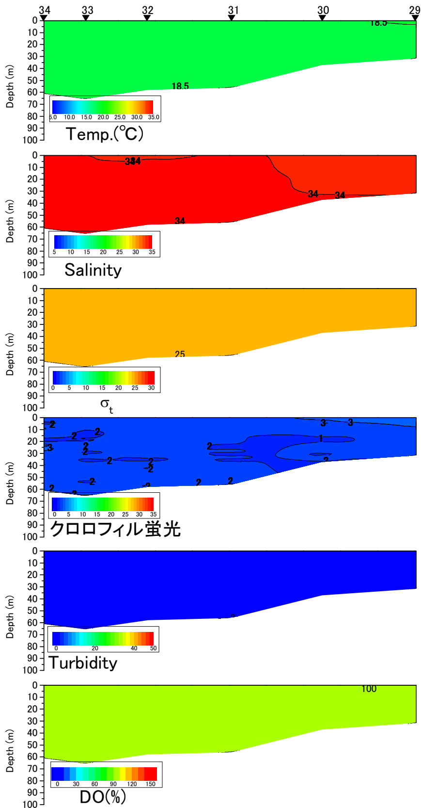
八代海西ラインの水温(°C)、塩分、密度( \sigma_t )、クロロフィル蛍光強度、濁度、溶存酸素飽和度(DO%)の鉛直面図(国土交通省の調査による) (2017年5月12日)
